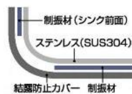
制振材により水音を 抑える静音仕様です。
